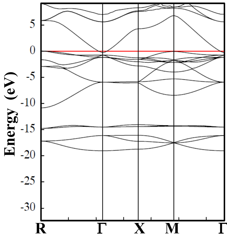
GGA (PBE96)
